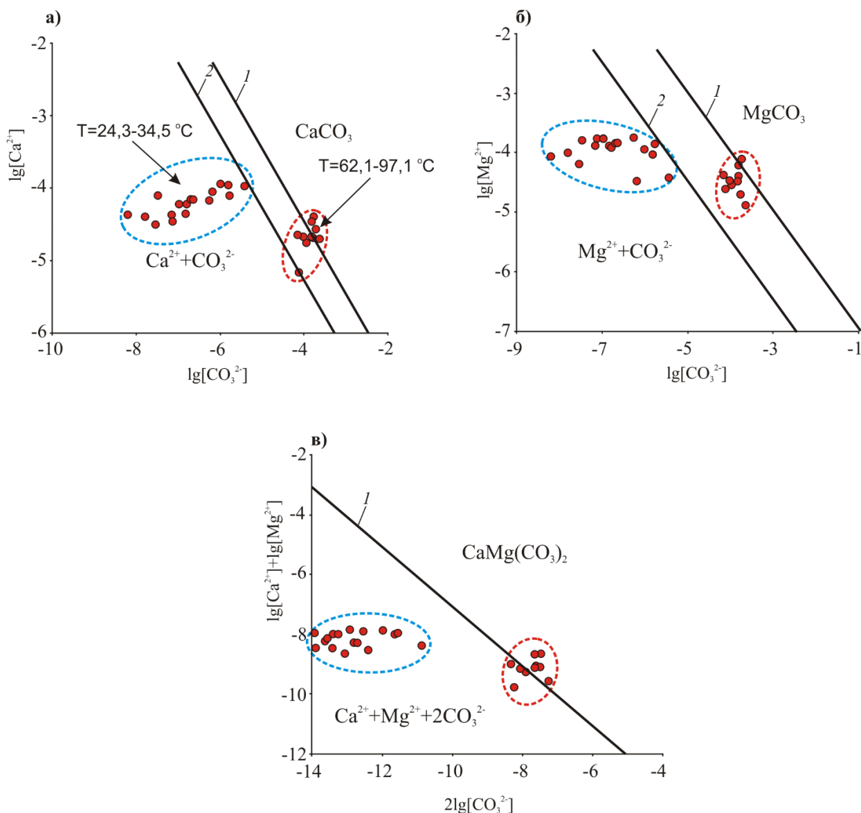
Рис. 3. Диаграммы степени насыщения термальных вод месторождения Банг кальцитом (а), магнезитом (б) и доломитом (в) при 25 °C (линия 1) и 100 °C (линия 2)
