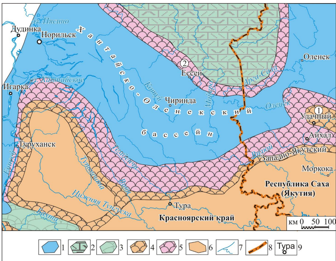
Палеогеографическая схема на майский век центральной части Сибирской платформы:
