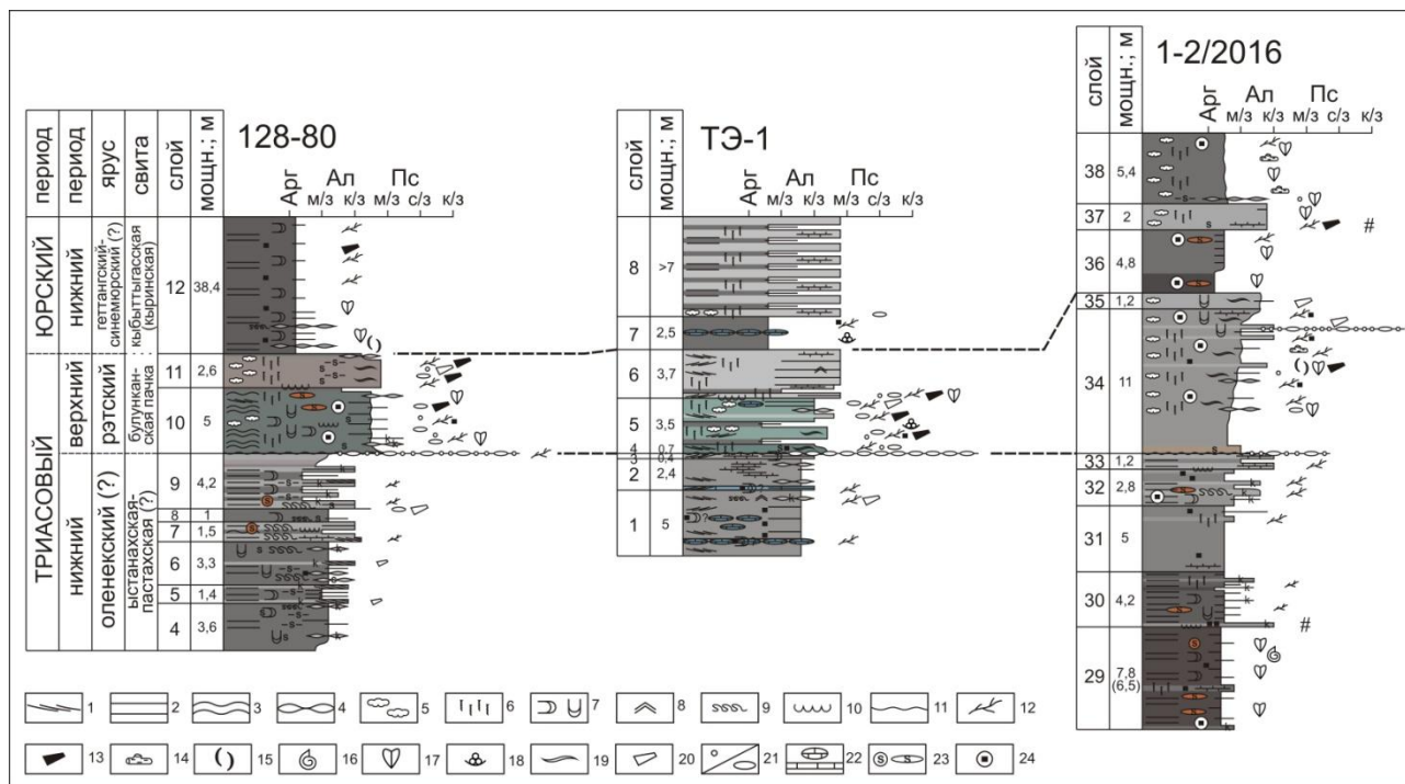
Рис. 2. Седиментационные разрезы пограничных триас-юрских отложений бассейна р. Экиит:
