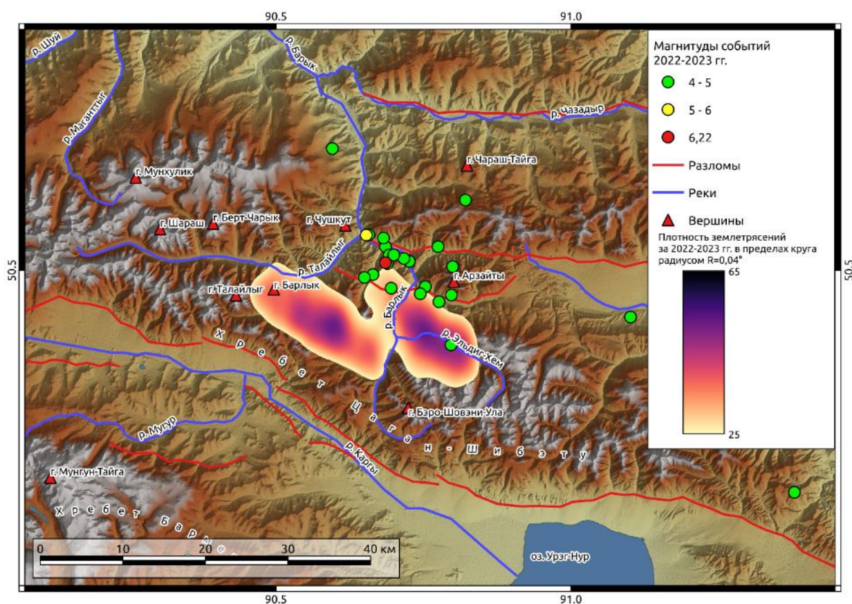
Рисунок 7 – Цаган-Шибэтинское землетрясение 29.07.2022 с M_L=6.2 и особенности сейсмичности его очаговой области за 2022-2023 гг.
