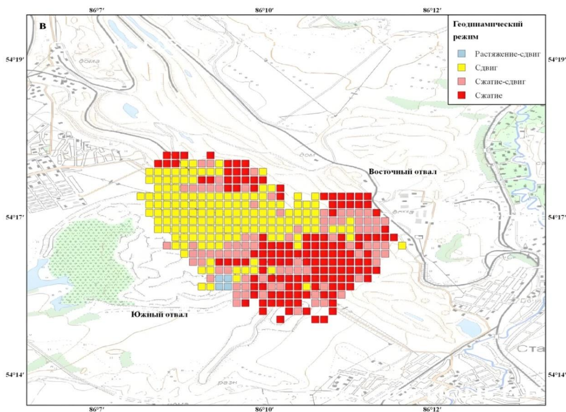
Рисунок 18 – Геодинамический тип напряженного состояния (желтый – горизонтальный сдвиг, красный – горизонтальное сжатие, светло красный – горизонтальный сдвиг со сжатием)
