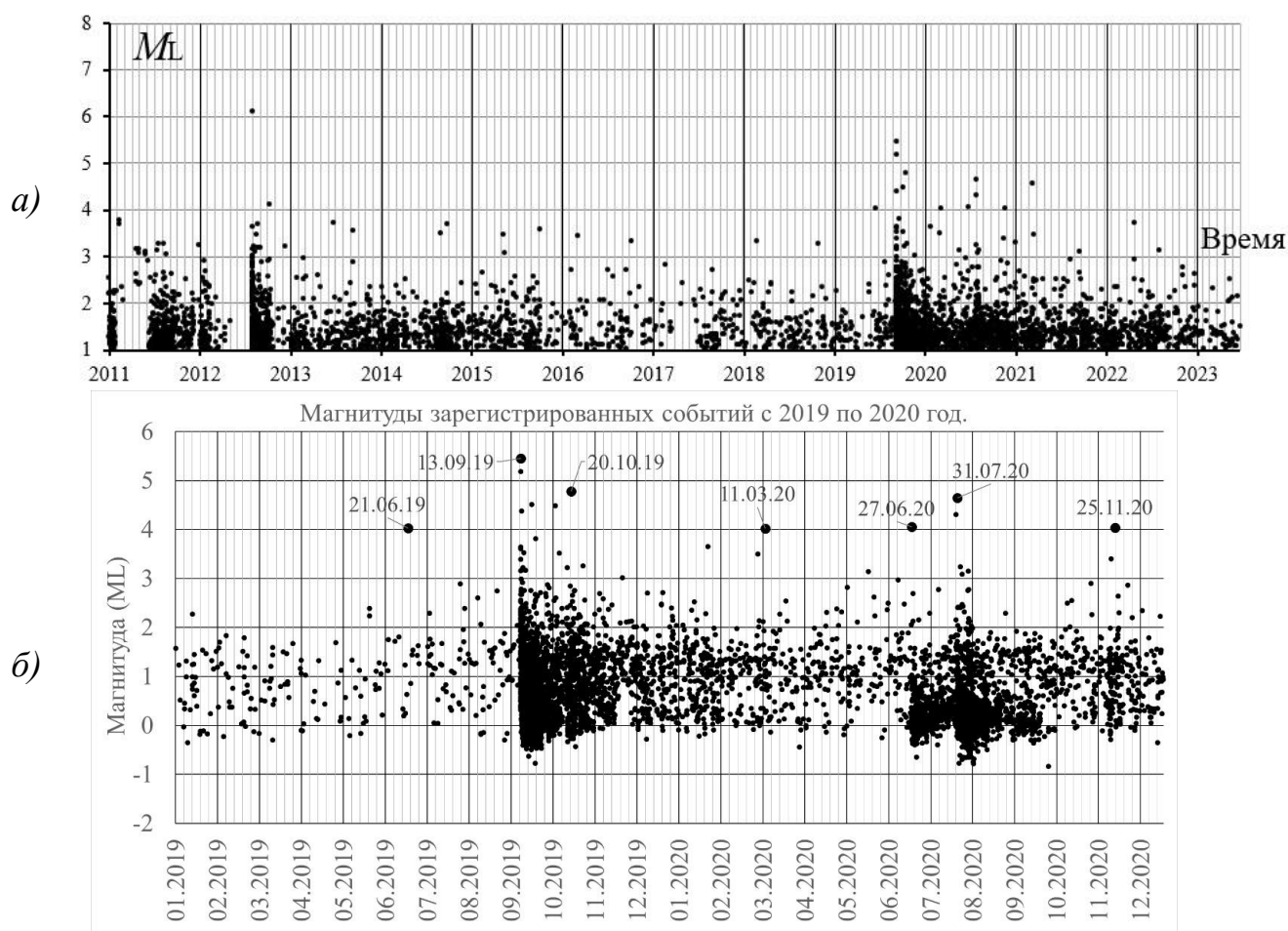
Рисунок 5 – Развитие сейсмического процесса в Айгулакской очаговой области. а – интервал с 2011 по 2023 гг., б – детальное рассмотрение интервала с 2019 по 2020 гг.
